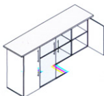
ARMÁRIO EXECUTIVO: cód.:100077- 2000 X 500 X 740
